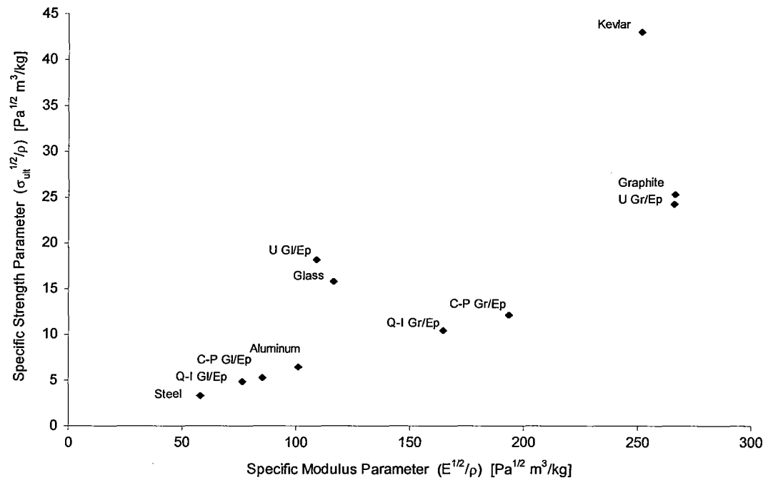
Specific Strength Parameter vs Specific Modulus Parameter
